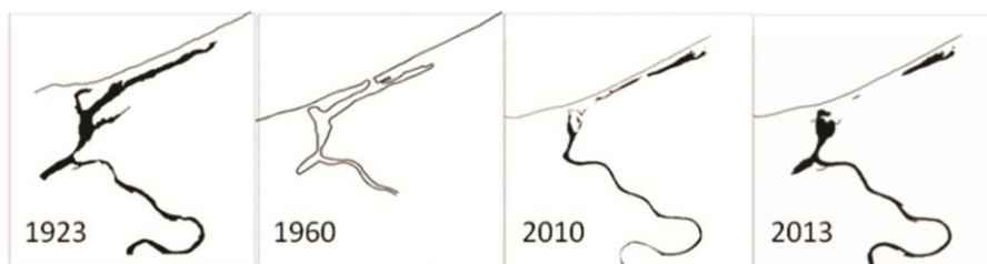
Figura 6: Evolución reciente de la desembocadura del estero El Yali y la Albufera. Fuente: Contreras y Figueroa (en preparación).
