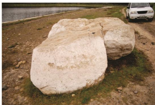
Figura 5.- Bloque de gneis representativo del basamento metamórfico situado en Laguna La Colejuda (33°45' 51" S - 71°42' 04" O) Fuente: fotografía del autor, agosto 2013.
